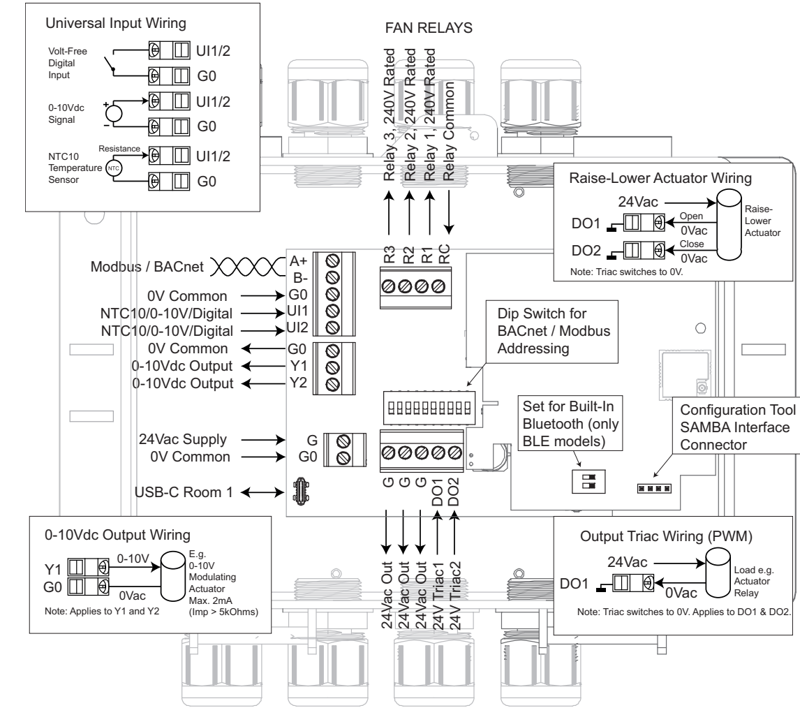
TCR83 WIRING
